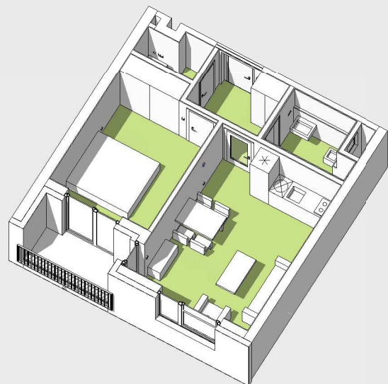
AXONOMETRIE
