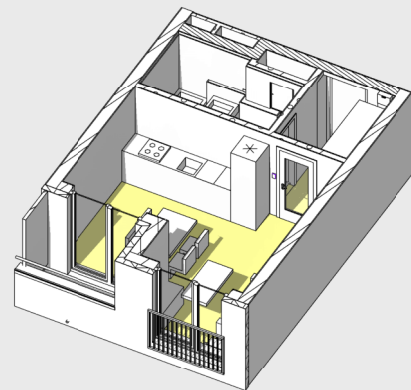
AXONOMETRIE
