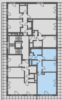
Půdorys podlaží
