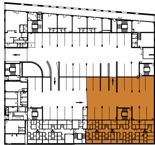
PŮDORYS PODLAŽÍ
