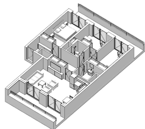
AXONOMETRIE BYTU
